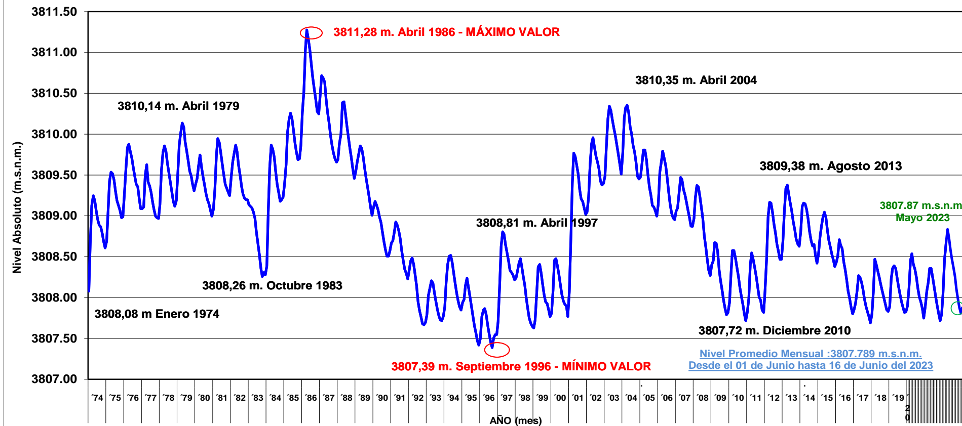
LAGO TITICACA: ESTACIÓN HUATAJATA NIVELES MEDIOS MENSUALES (SERIE 1974 - 2023)
